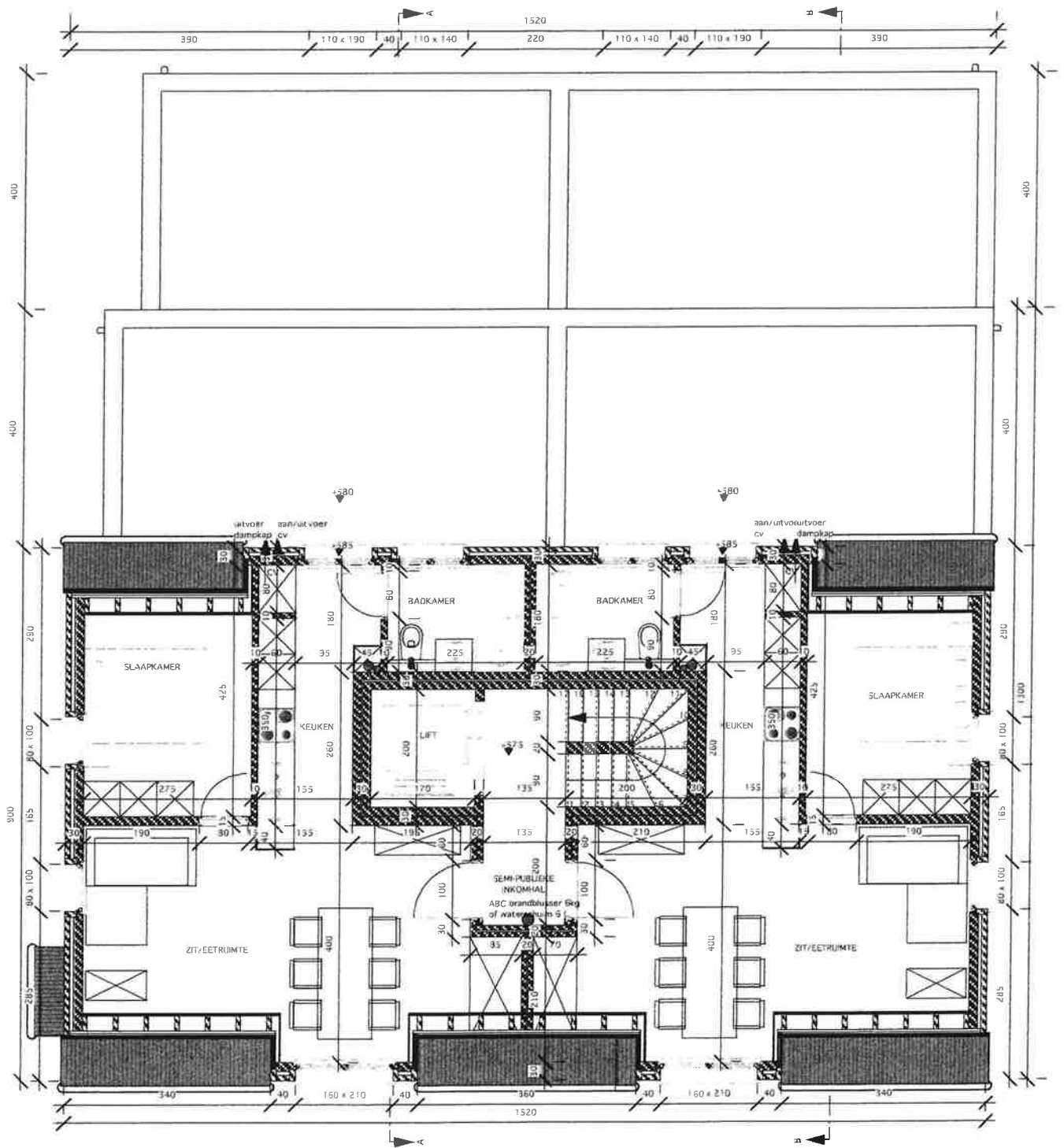
Verdiepingsplan 2 schaal: 1/100
